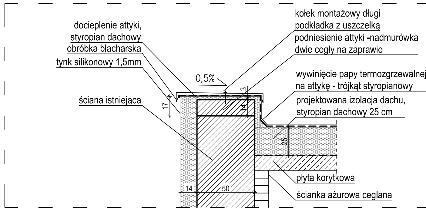
D2 - detal podwyższenia attyki
