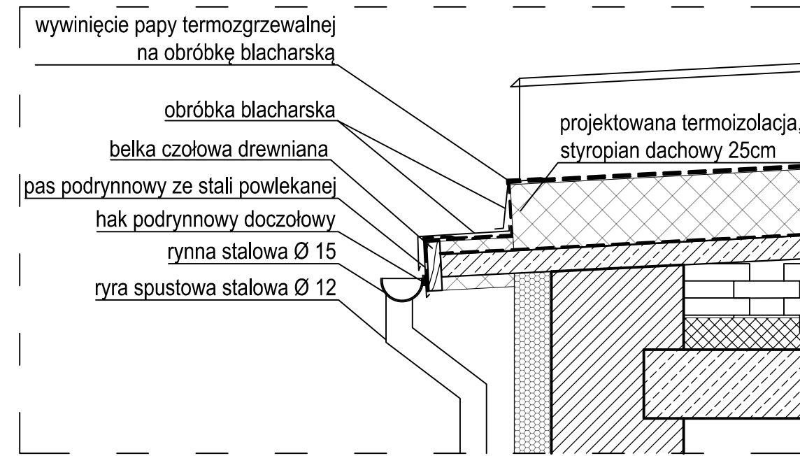
D1 - detal mocowania rynny
